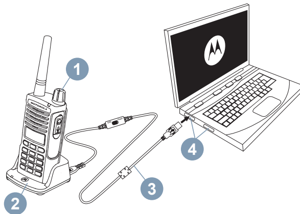
Kuva 1: Radiopuhelimen asentaminen CPS-ohjelmiston avulla
