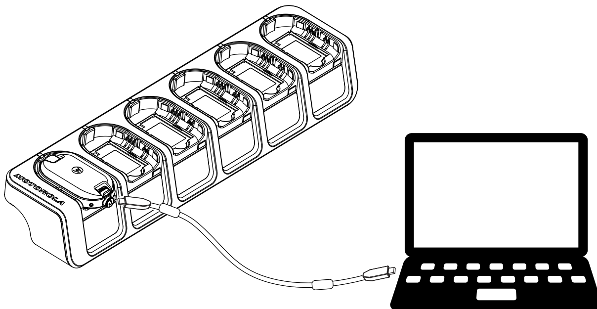
Рисунок 11: Программирование радиостанции с помощью многоместного зарядного устройства
