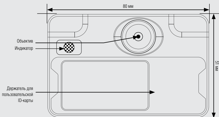
Вид спереди
