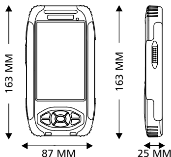
Вид спереди
