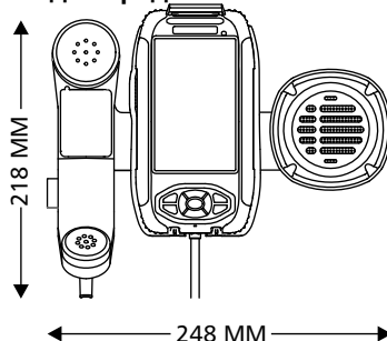
Вид спереди
