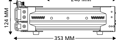
Вид сбоку
