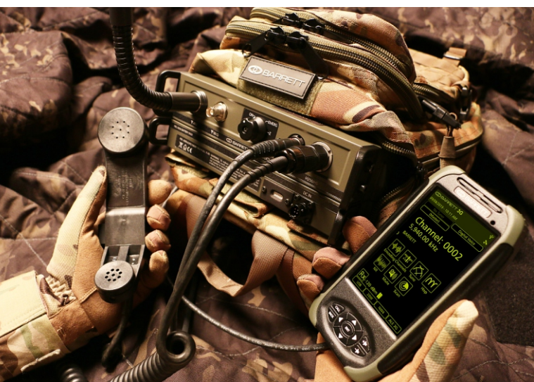
Barrett PRC-4090 HF SDR manpack avec sac à dos multicam et combiné H250 optionnel.
